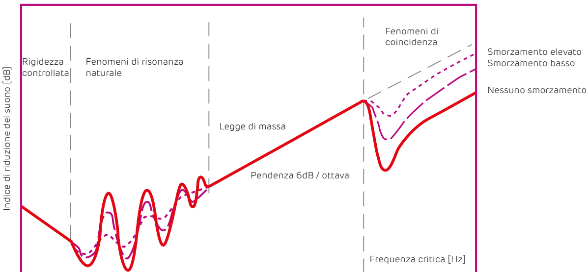
Fig. 14 - Campo di validità della legge della massa
