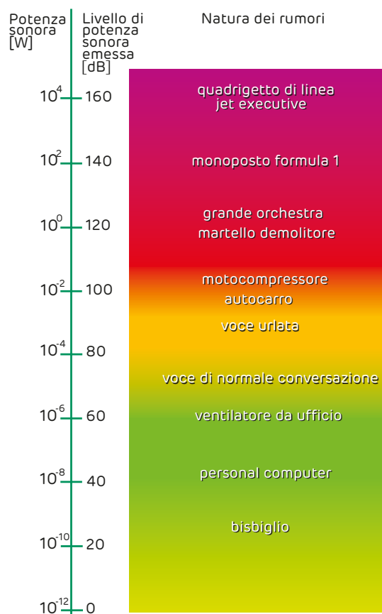
Fig. 6 - Livello di potenza sonora emessa da alcune macchine
