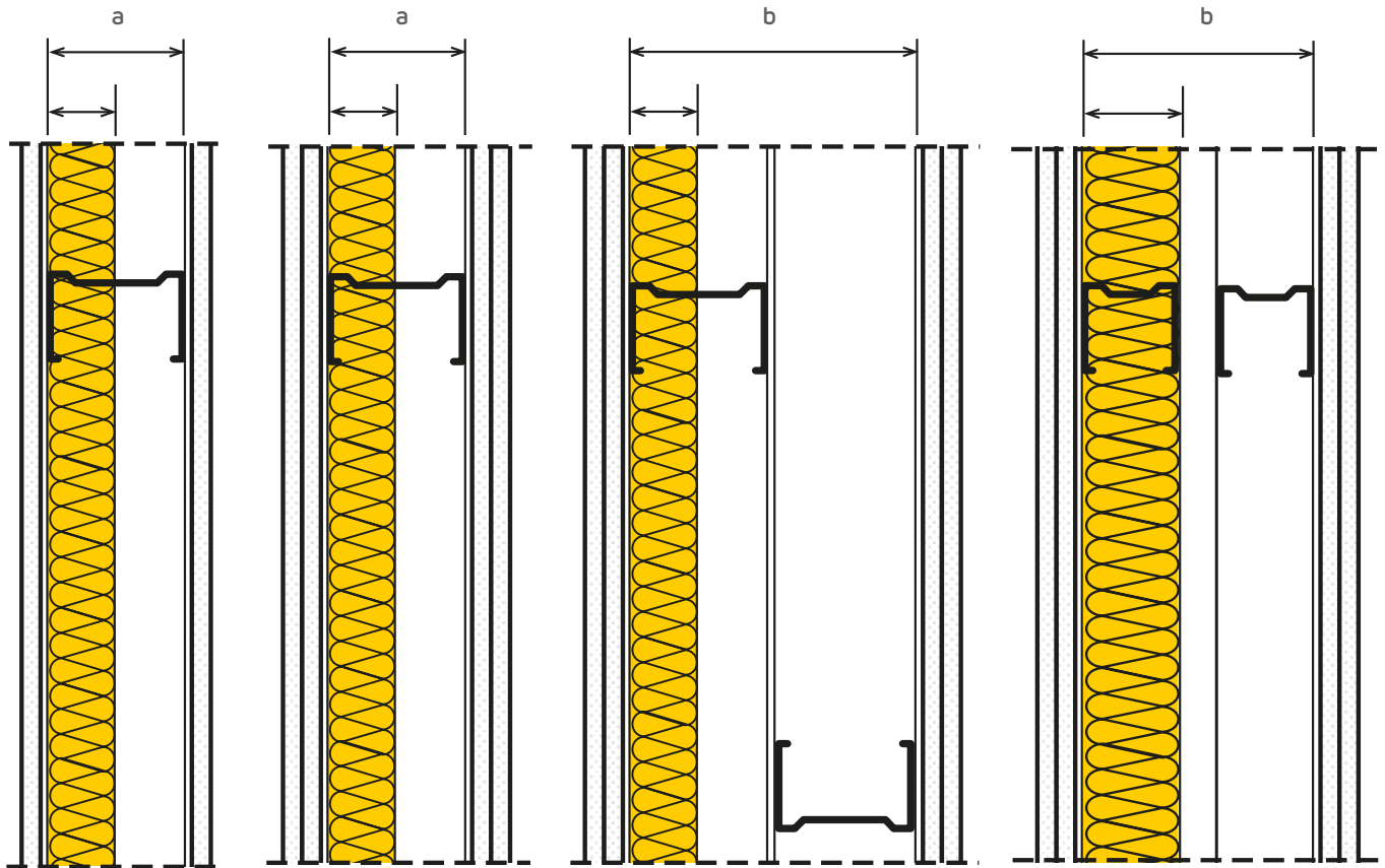
Fig. 30 - Sistemi ad orditura semplice (a) e ad orditura doppia (b)
