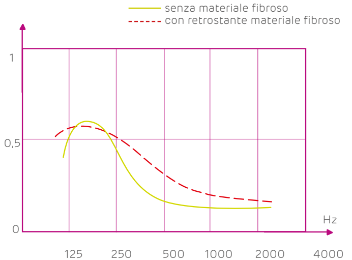
Fig. 17 - Assorbimento per risonanza di membrana
