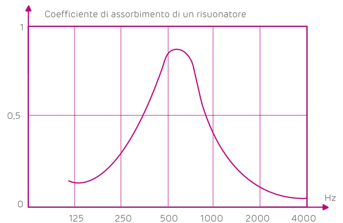
Fig. 16 -Assorbimento per risonanza di cavità
