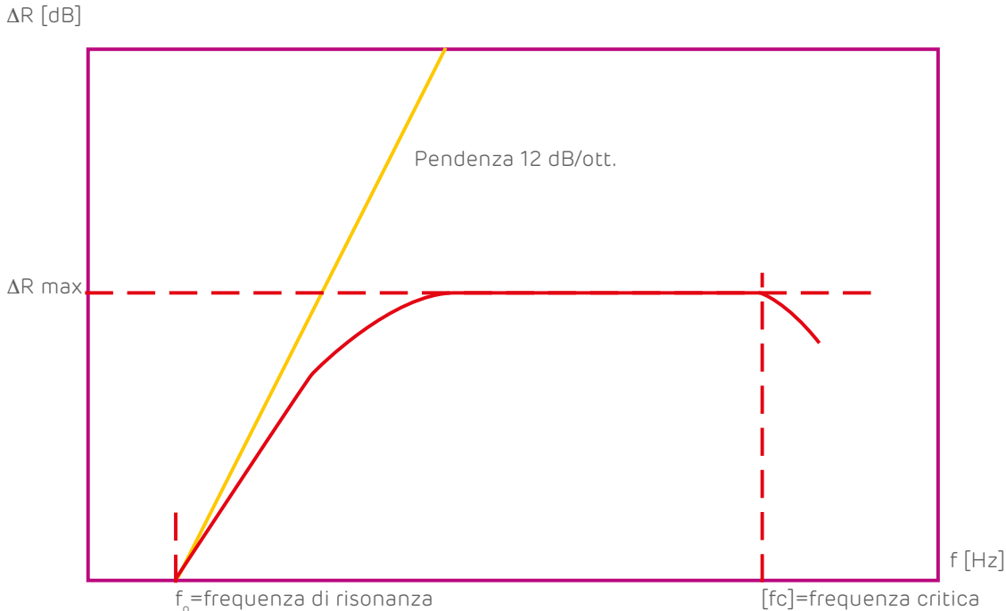
Fig. 33 - Miglioramento \Delta R del potere fonoisolante grazie all'impegno di una controparete
