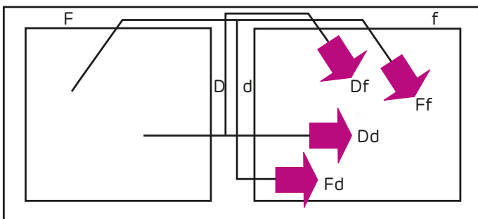
Figura 37: Indicazione dei percorsi delle trasmissioni diretta e laterale di rumori aerei
