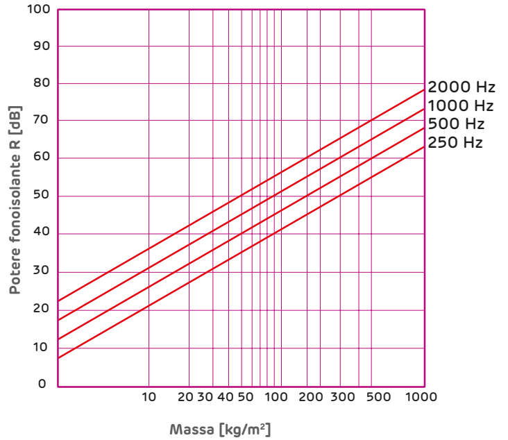
Fig. 13 - Rappresentazione schematica della legge della massa
