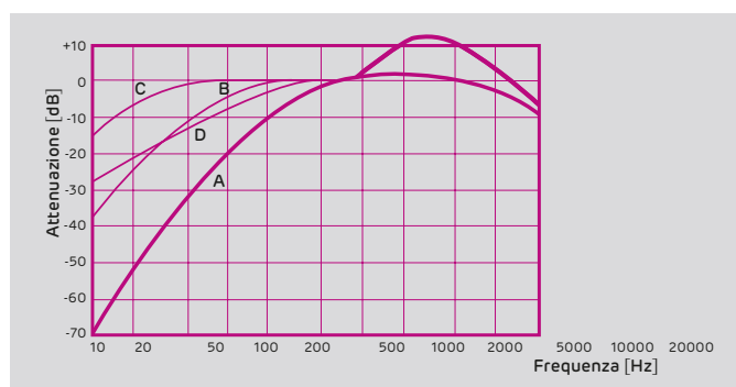
Fig. 9 - Curve di ponderazione
