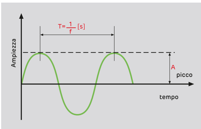
Fig.3 - Pressione sonora in funzione del tempo (fenomeno sinusoidale)
