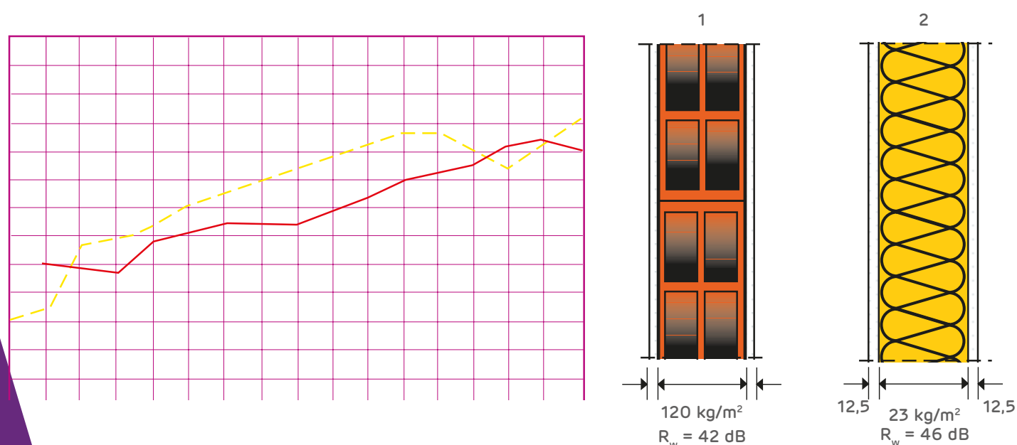
Fig. 27 - Confronto tra il potere fonoisolante di una parete in muratura e di un divisorio di lastre in gesso rivestito
