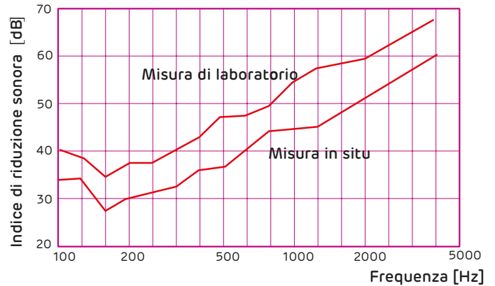
Fig. 21 - Indice di valutazione del potere fonoisolante misurato in laboratorio e in opera per una muratura di calcestruzzo di spessore 15 cm
