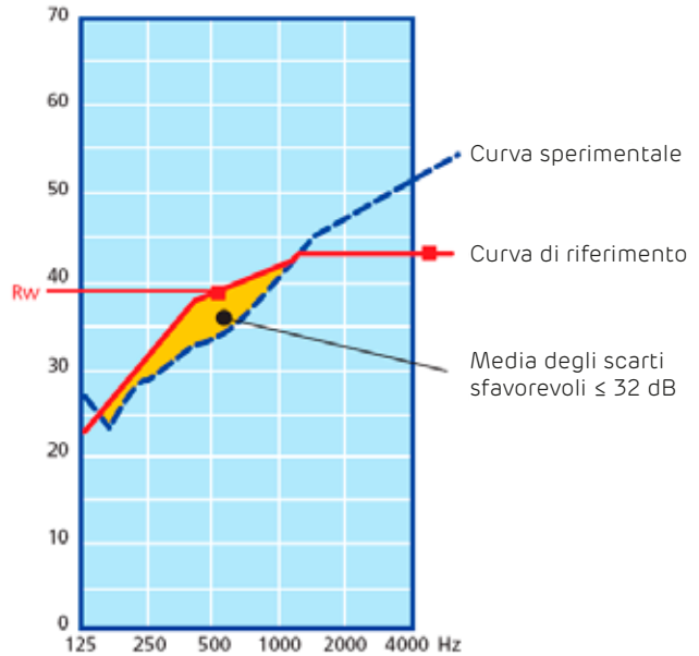
Fig. 20 - Indice di valutazione del potere fonoisolante R_w
