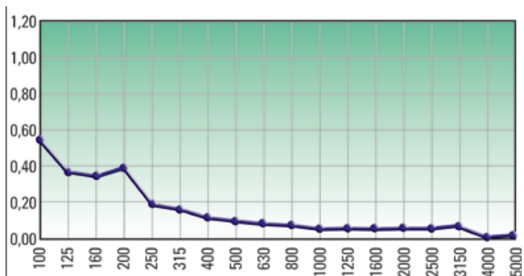
Fig. 35 - Assorbimento acustico lastra cieca di cartongesso con interposto strato di lana di vetro di spessore 80 mm e massa volumica 20 Kg/m 3 - Plenum da 100 mm
