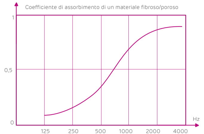
Fig. 15 -Assorbimento per porosità
