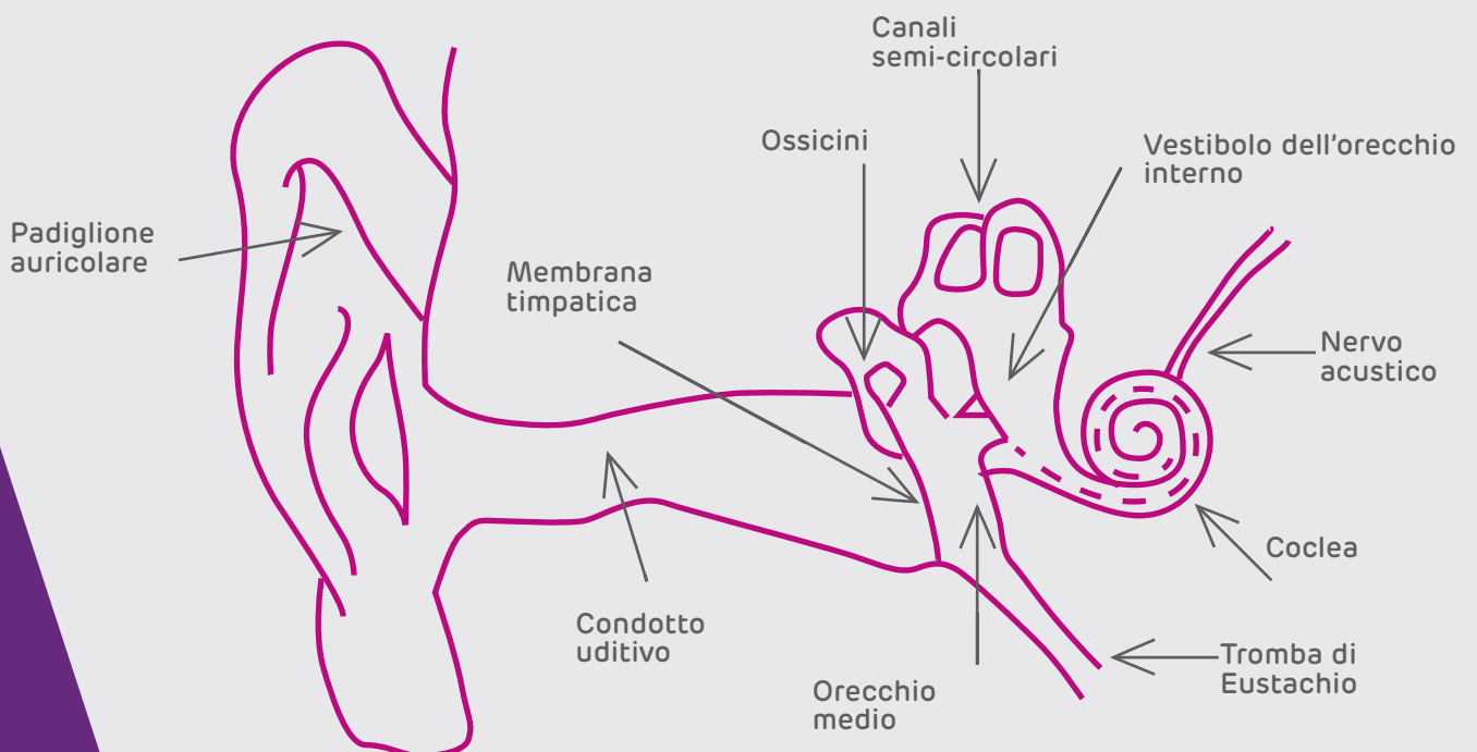
Fig. 7 - Apparato uditivo
