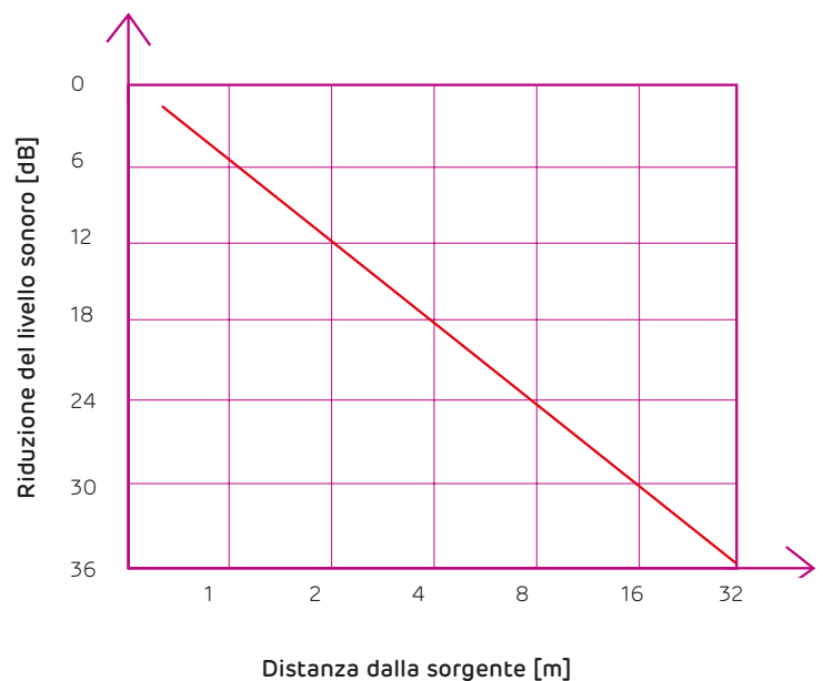
Fig. 10 - Riduzione del livello di pressione sonora in funzione della distanza dalla sorgente
