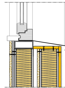
Giunto infisso – sezione verticale
